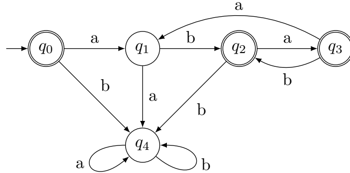
Figura 1.1: Exemple de representació d'autòmat determinista
