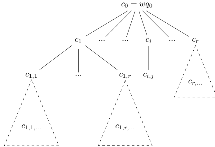
Figura 2.1: Esquema d'un arbre de còmputos
